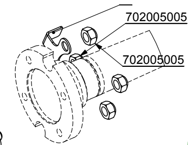
DÉTAIL A ECHELLE 1 : 3
