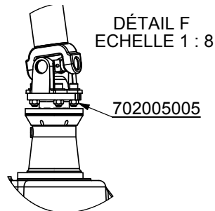
MONTAGE ECROU DEFORME SUR ARBRE DE BOITE
