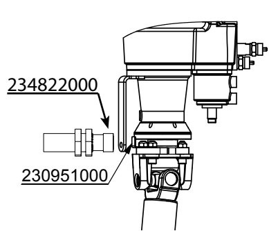
Capteur vitesse / Speed Sensor 234822000
